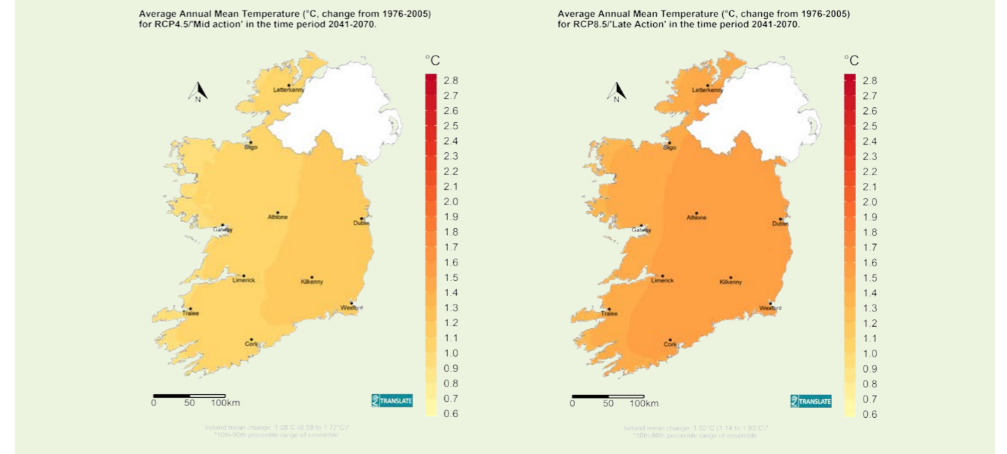
Fíor 29 Samhaltú bunaithe ar athrú Mheánteocht Airmheánach Met Éireann i gcoibhneas le bunlíne 1976-2005 don tréimhse idir 2041-70 faoi chás CCC4.5 agus CCC8.5.
