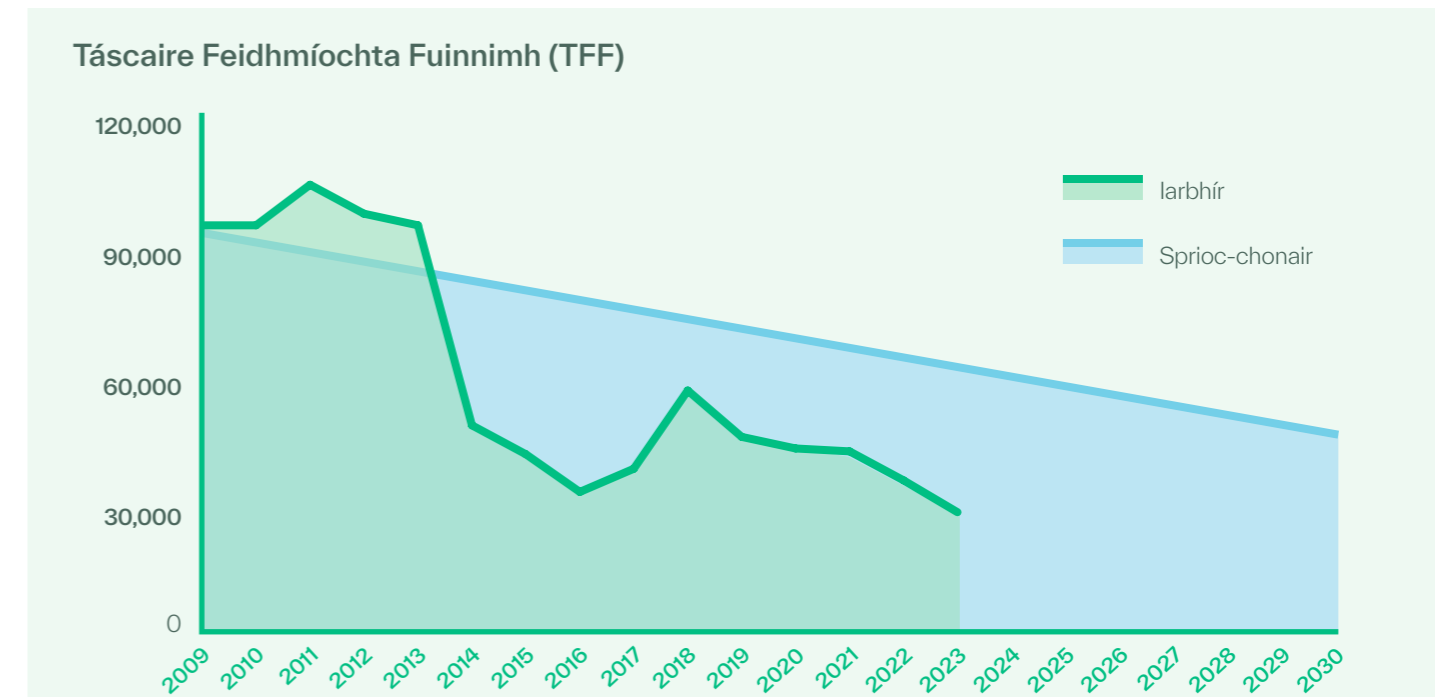
Fíor 2 Sonraí SEAI a léiríonn Táscaire Feidhmíochta Fuinnimh (EnPI) Bhord na Móna idir 2009–2023]
